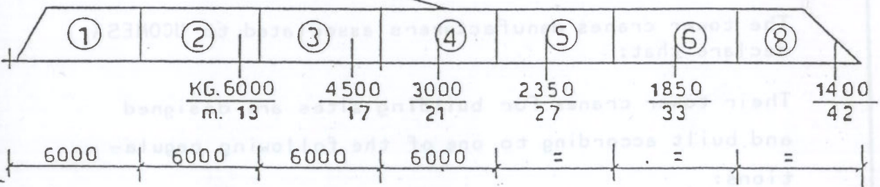
JIB 42 mt.
