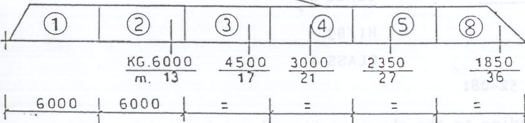
JIB 36 mt.
