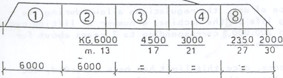
JIB 30 mt.
